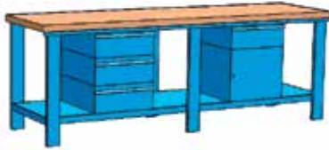
● MG 108/BC Banco dotato di 1 cassetiera MG 117 e 1 cassetiera MG 118 Bench with 1 chest of drawers MG 117 and 1 MG 118 | Etabli avec caisson MG 117 et caisson MG 118
