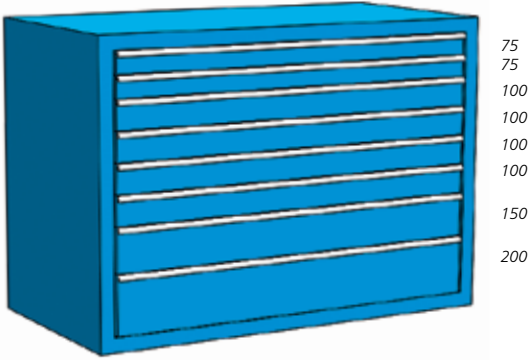
● h. 1000 mm • 8 cassetti V100 85T estrazione totale 200 kg
