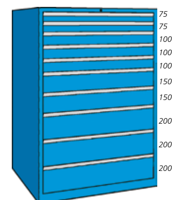
● h. 1450 mm • 10 cassetti B145 02 estrazione parziale B145 02T estrazione totale 200 kg B145 02V estrazione totale 75 kg
