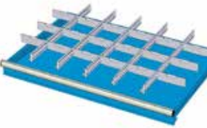
5 divisori fessurati 36 U 18 divisori trasversali 9 U SD 5013 per cassetti da 50 mm SD 7515 per cassetti da 75 mm SD 10016 per cassetti da 100-125 mm SD 15016 per cassetti da 150 mm SD 20015 per cassetti da 200 mm SD 30010 per cassetti da 300 mm
