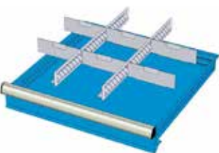
2 divisori fessurati 27 U 6 divisori trasversali 9 U SD 5026 per cassetti da 50 mm SD 7532 per cassetti da 75 mm SD 10033 per cassetti da 100-125 mm SD 15033 per cassetti da 150 mm SD 20025 per cassetti da 200 mm SD 30016 per cassetti da 300 mm
