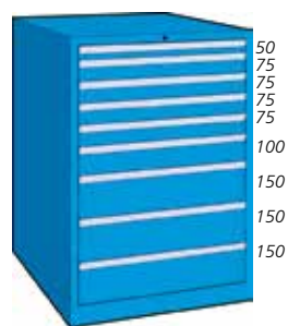
● h. 1000 mm • 9 cassetti M100 94 estrazione parziale M100 94T estrazione totale 200 kg M100 94V estrazione totale 75 kg
