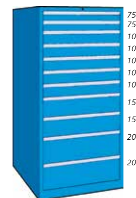
● h. 1450 mm • 11 cassetti M145 111 estrazione parziale M145 111T estrazione totale 200 kg M145 111V estrazione totale 75 kg
